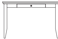
Desk (1 drawer) 1951001 D24xW48xH31 1951002 D26xW48xH31 1951003 D28xW48xH31 1951004 D30xW48xH31 1951005 D28xW54xH31 1951006 D30xW54xH31
